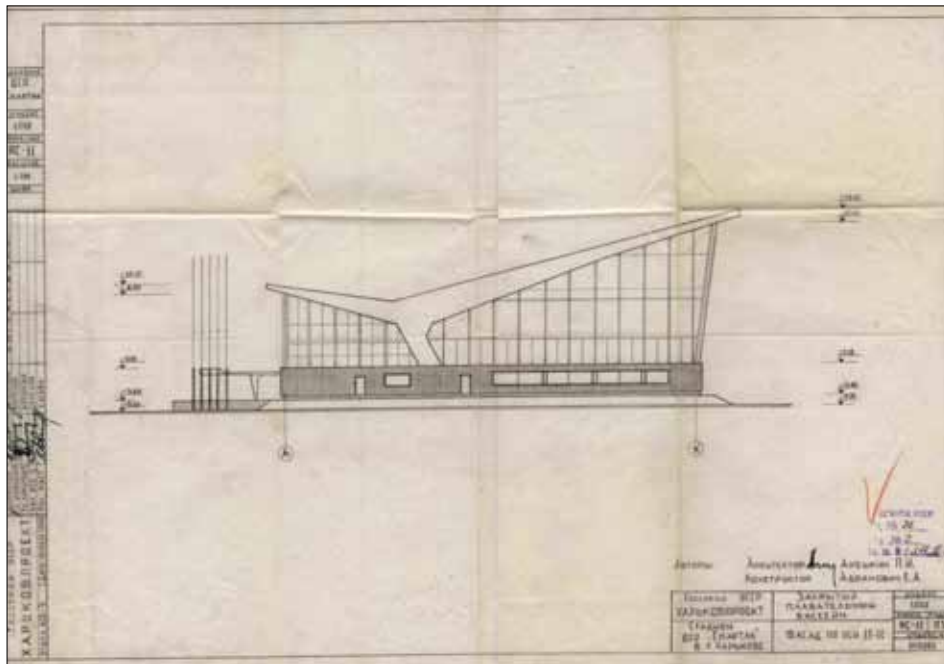
Закритий плавальний басейн на стадіоні Спартак у м. Харкові. Фасад. 1966 р.
