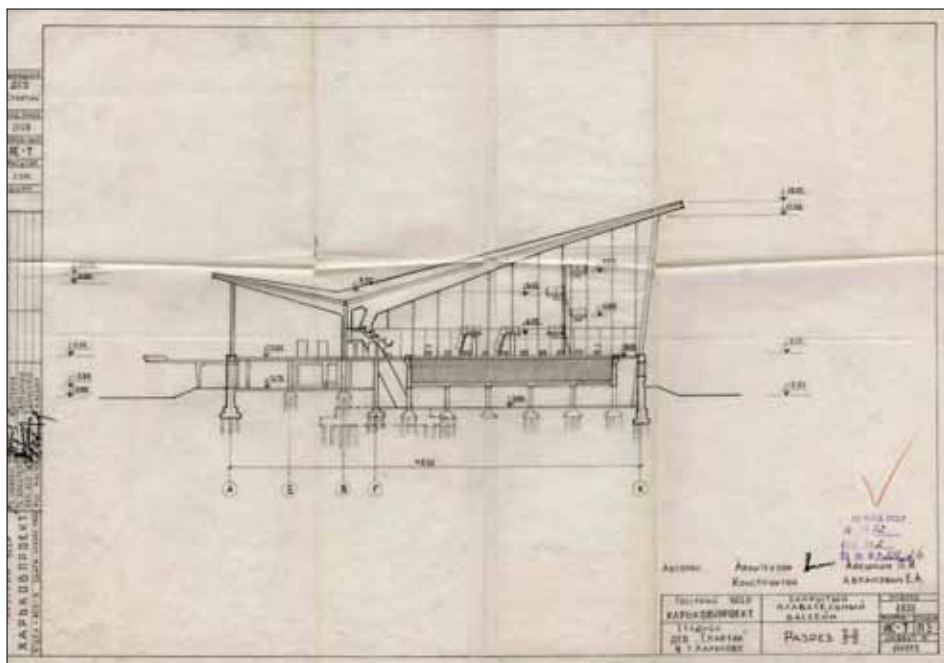
Закритий плавальний басейн на стадіоні Спартак у м. Харкові. Розріз. 1966 р.
